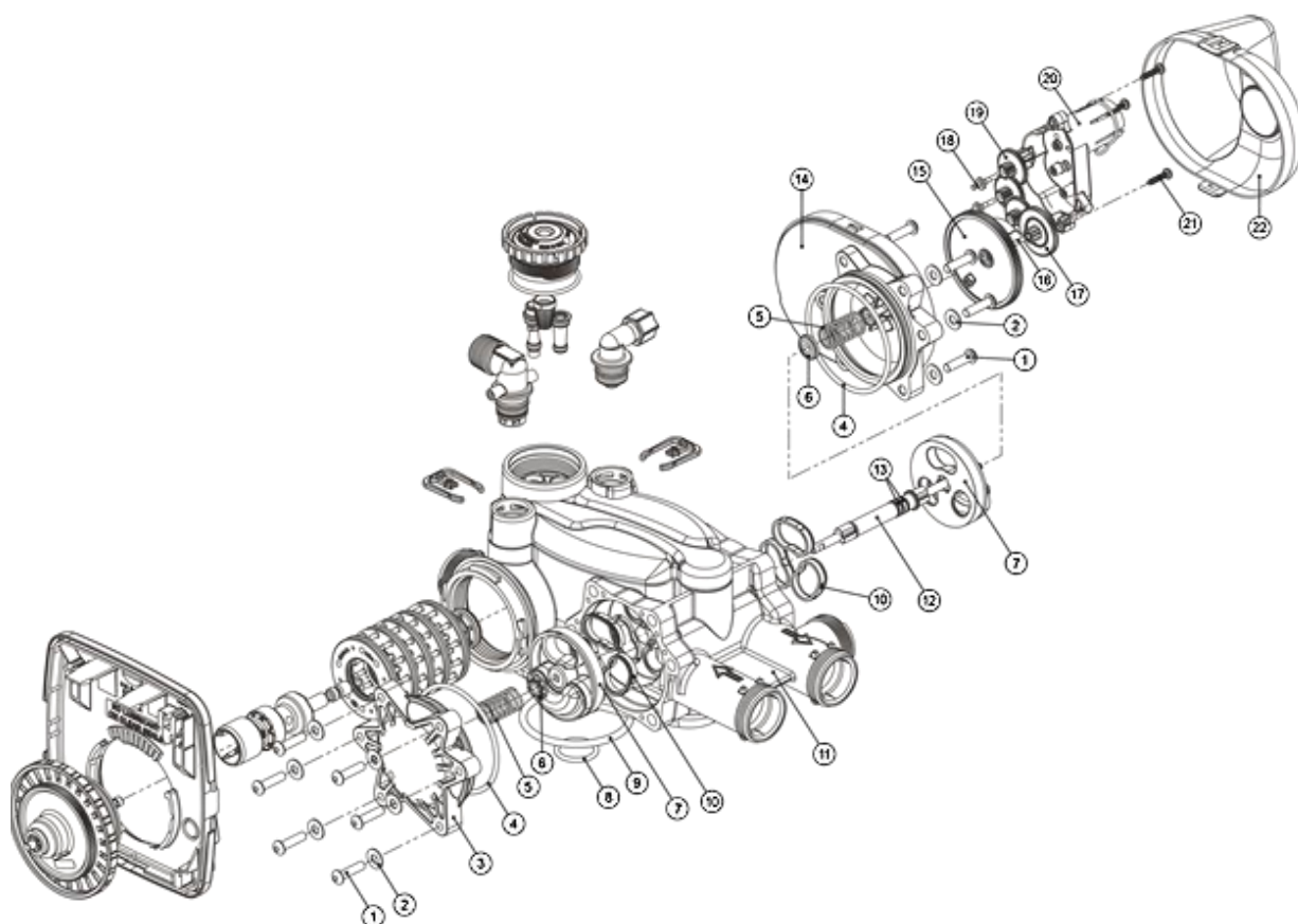
Bild 12. Ersatzteile für Steuerventil WS 1 CI Twin-Twin
