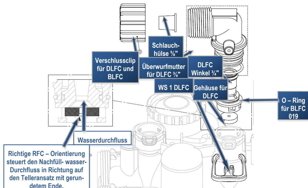
Bild 8. Abwasserblendeneinheit( \frac{3}{4} ").
