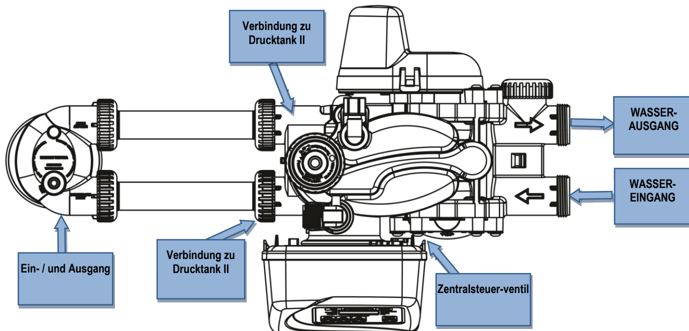
Bild 3. Steuerventil WS 1 CK Twin-Twin - Draufsicht
