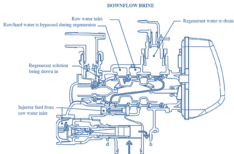
Bild 19. Betriebszyklen der Enthärtungsanlage – dn Besalzen
