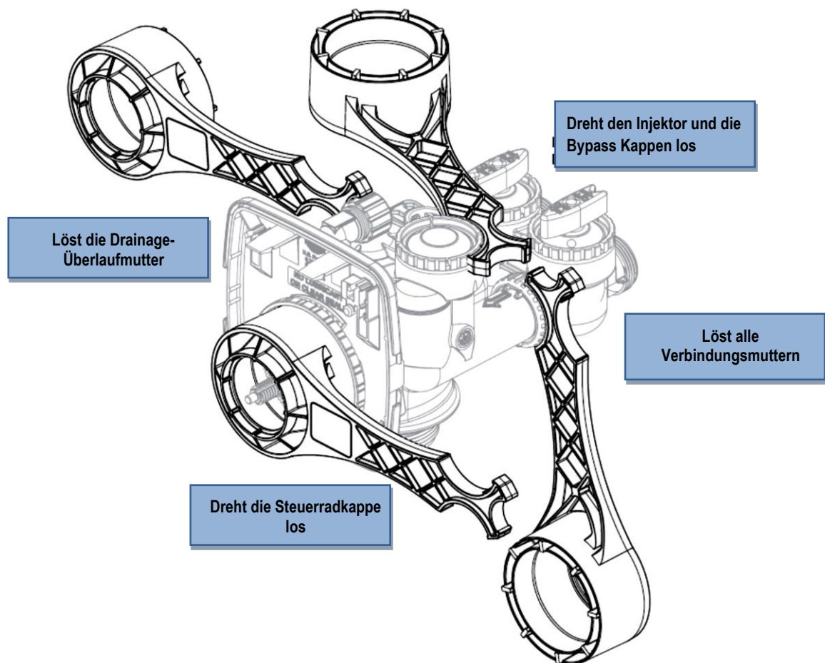
Bild 15. WS1 – Montageschlüssel.
