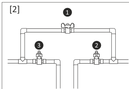
ПОЛОЖЕНИЕ ОБВОДА [2]
