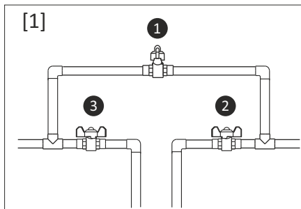
РАБОЧЕЕ ПОЛОЖЕНИЕ [1]
