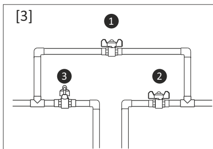
ПОЛОЖЕНИЕ ОБСЛУЖИВАНИЯ [3]
