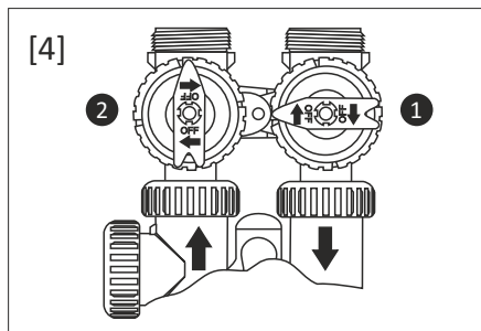
ЗАКРЫТОЕ ПОЛОЖЕНИЕ [4]
