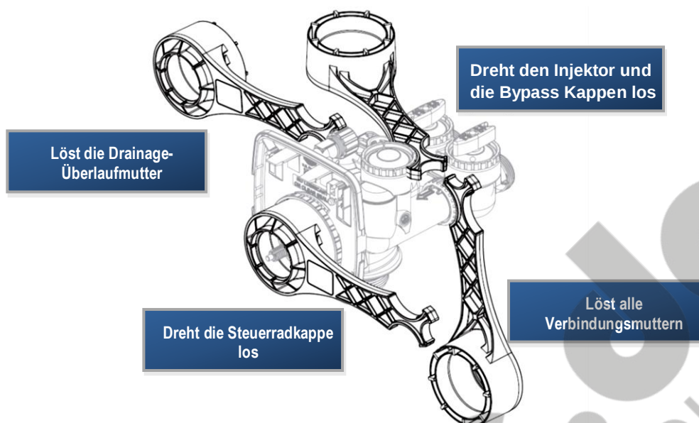
Bild 2. WS1 – Montageschlüssel.
