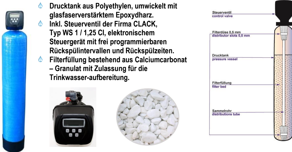
Bild 1. Bestandteile der CC-Filteranlage CC CI 1" / CC CI 1,25"
