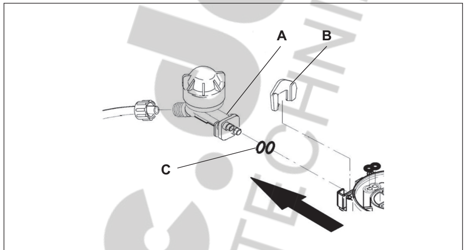
Abb. 17: Injektorbaugruppe abziehen
