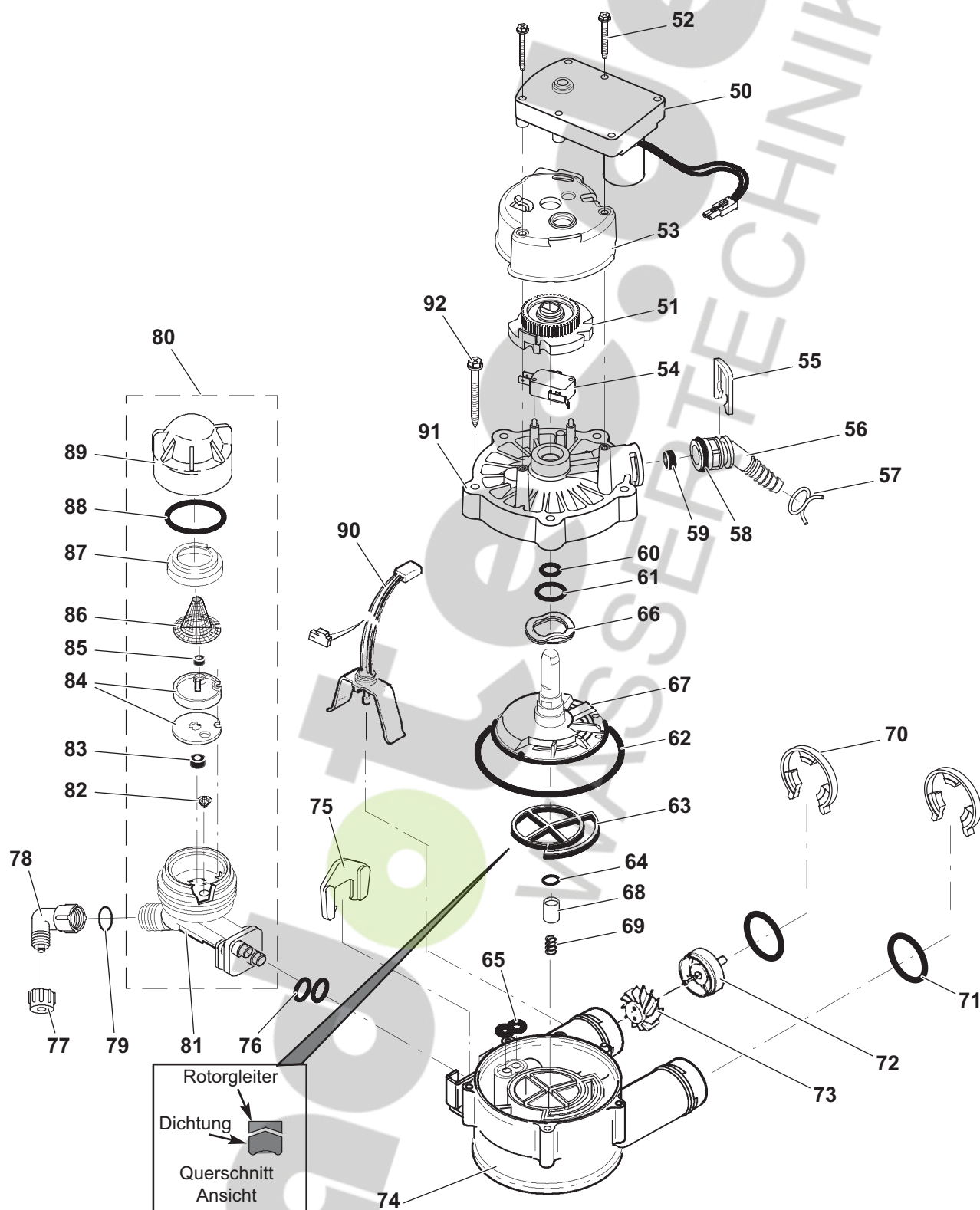
Abb. 25: Ventilbaugruppe
