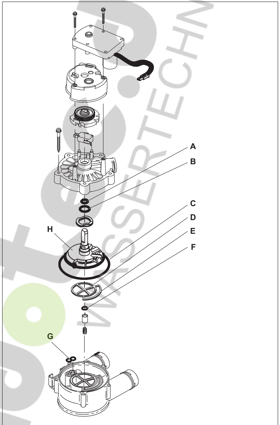
Abb. 15: Ventilbaugruppe
